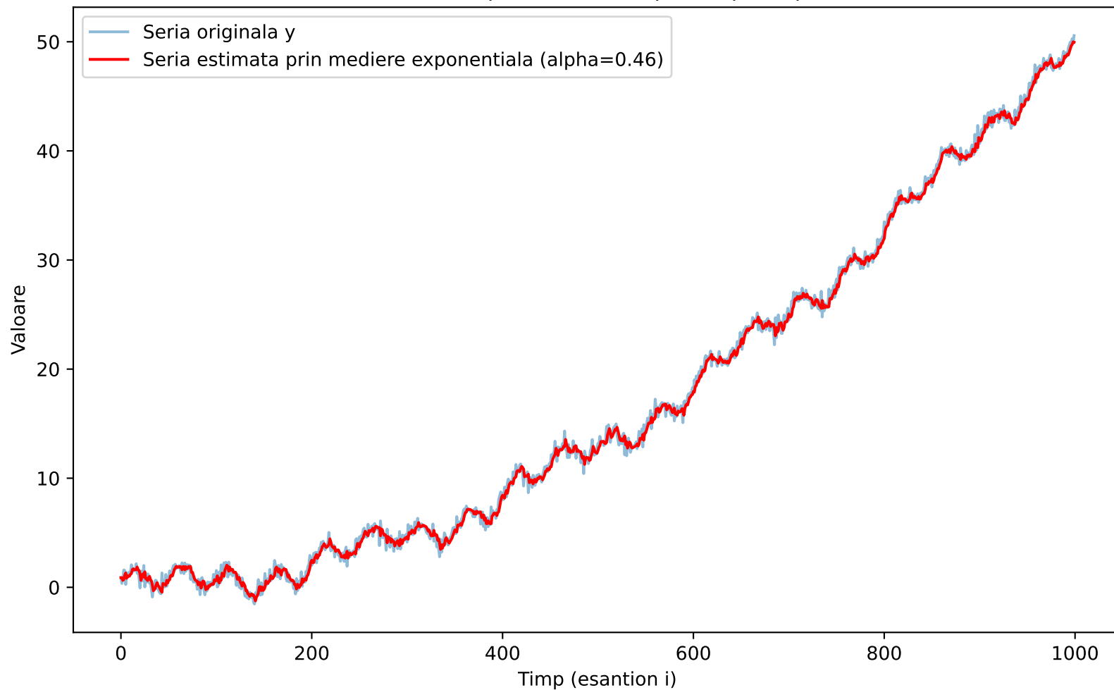
Medierea exponentiala simpla - alpha optim
